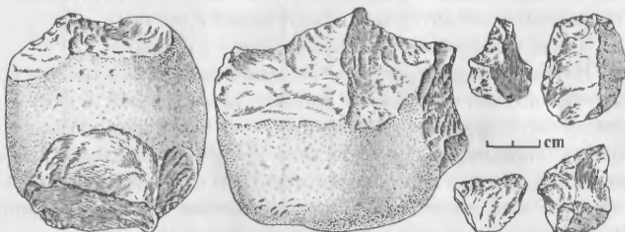
Рис. 8. Орудия олдувая*
