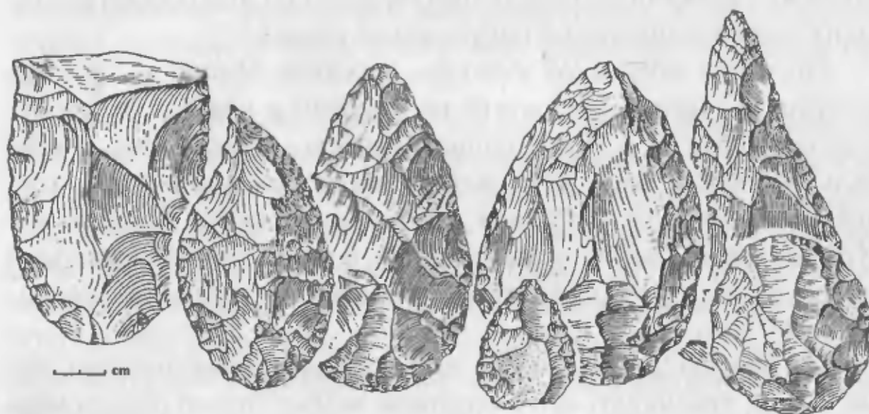
Рис. 7. Орудия ашеля**
