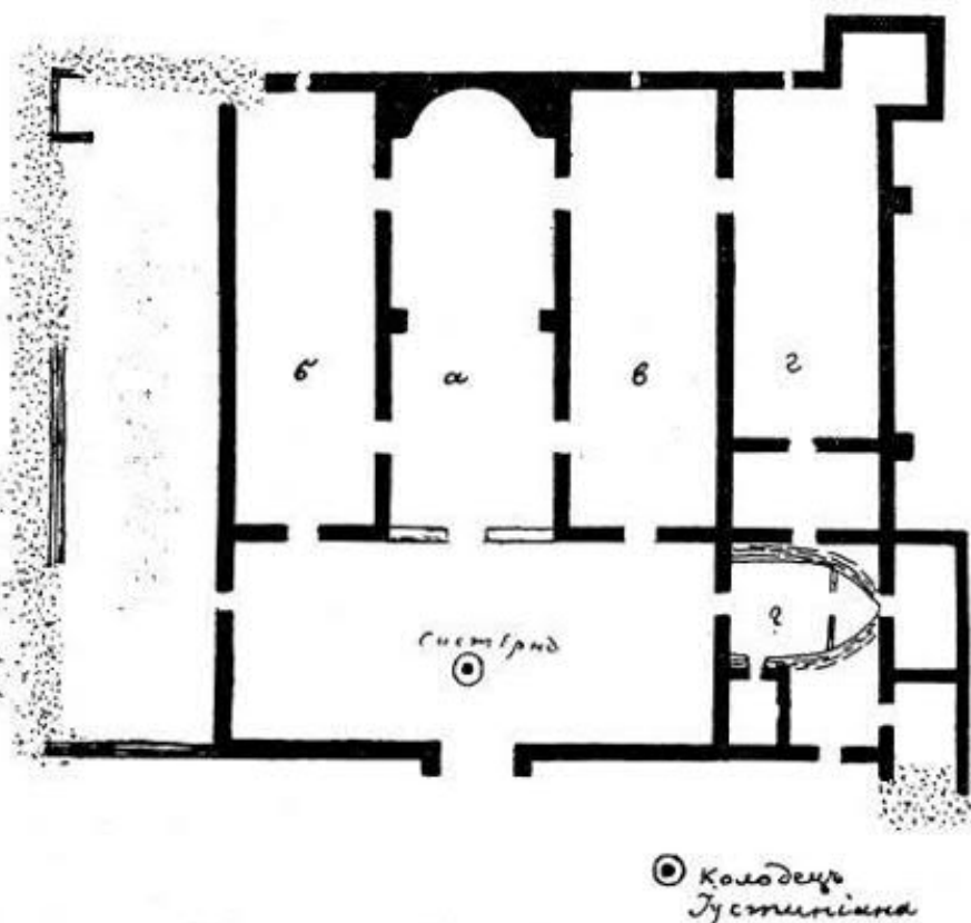
Планъ монастыря Іоанна Предтечи у Іордана.
