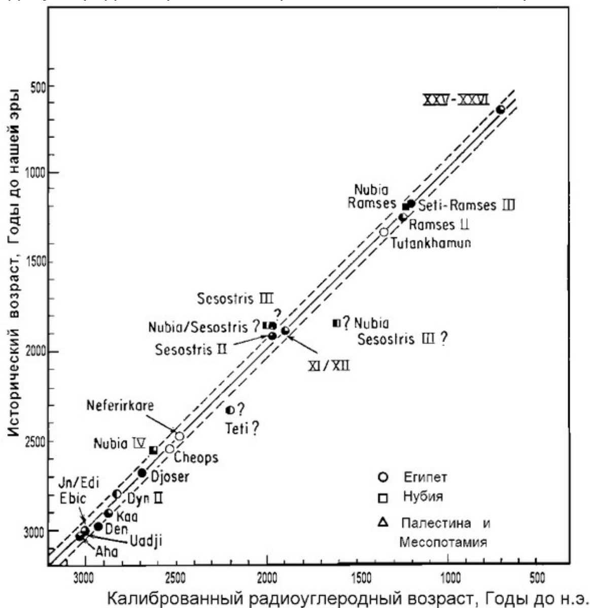
Рис. 6. Усредненные радиоуглеродные даты для исторических образцов из Египта, Нубии, Месопотамии и
