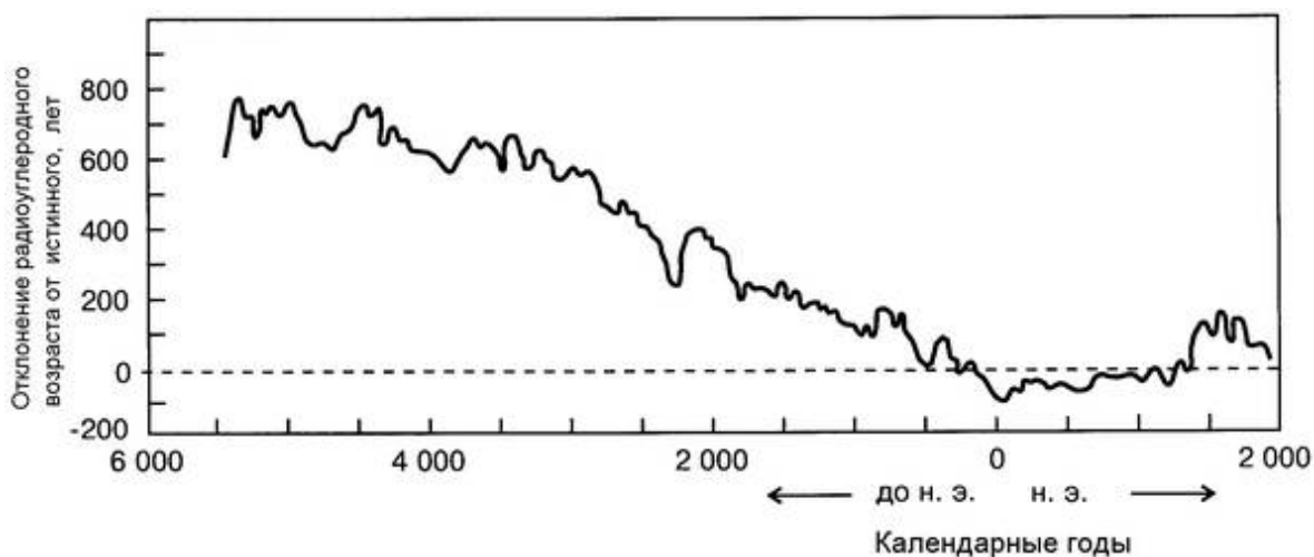
Рис. 5. Радиоуглеродная калибровочная кривая (радиоуглеродный возраст, годы BP), полученная датированием колец деревьев (календарные годы, BC/AD). Прямая линия означает равенство “радиоуглеродного” возраста абсолютному возрасту образцов ( ^{14}\text{C} годы = дендрогодам).
