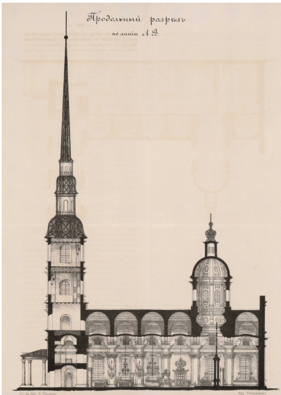
Продольный разрез
