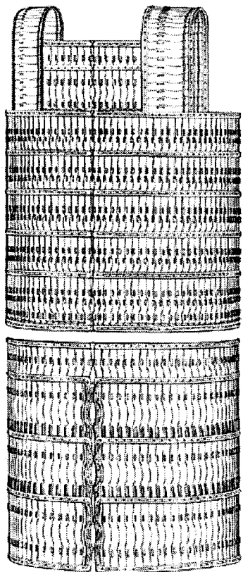
Реконструкция кочевнического пластинчатого доспеха из погребения 12 из Нидерштоттингена (Paulsen, 1967. Taf. 22): верхняя часть — для защиты груди, нижняя, с разрезами спереди и сзади, — для защиты бедер сидящего в седле воина
