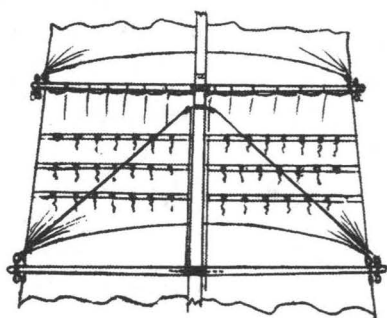
Прямой парус
